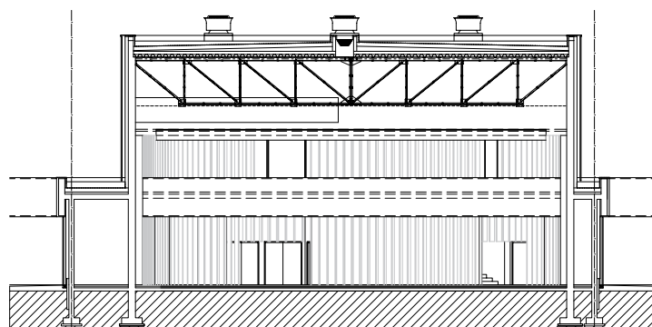
Rez celým komplexom a rez viacúčelovou sálou
