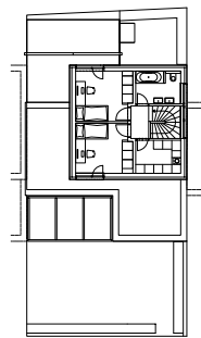
Pôdorys 2. np
