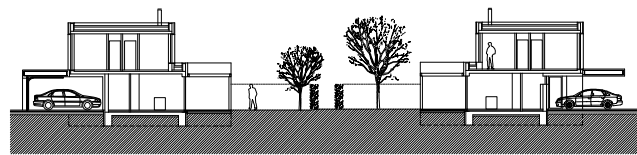
Rez pozdĺžny
